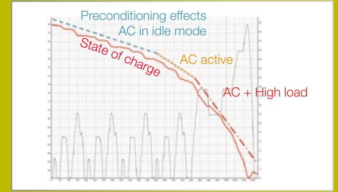
バッテリー残量のトラッキング
