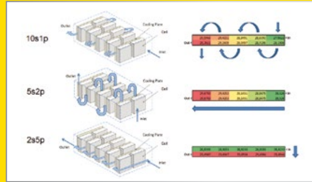
バッテリーパッケージ/バッテリーセルの熱管理
